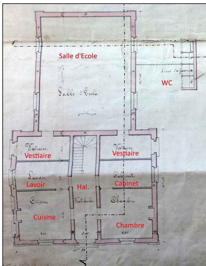
3: Gelijkvloers. Bovenaan het schoolgedeelte en onderaan het woonhuis. Plan uit 1865.
