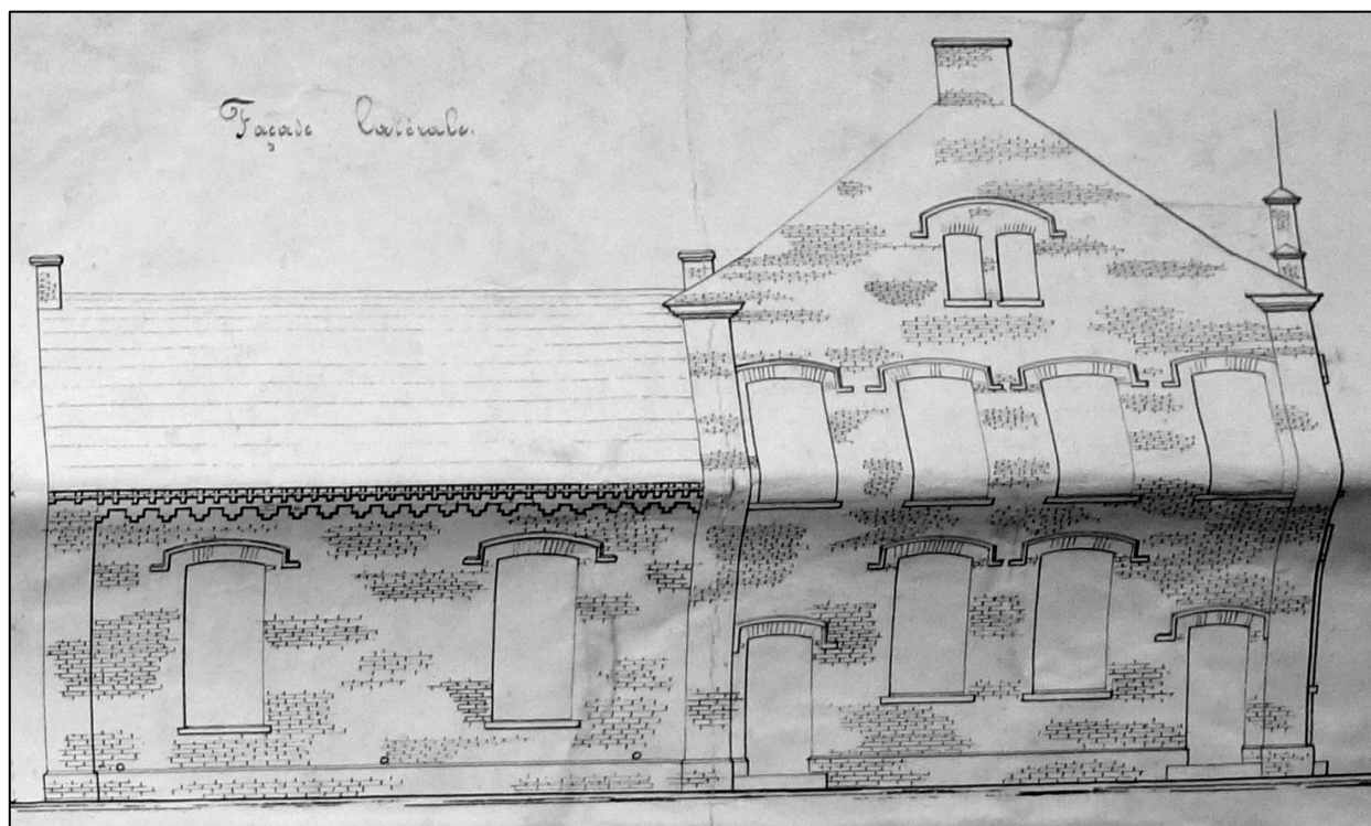
6: Gevel langs de kant van de Molenstraat
